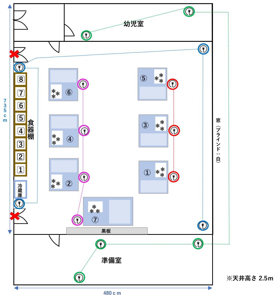
配置図
